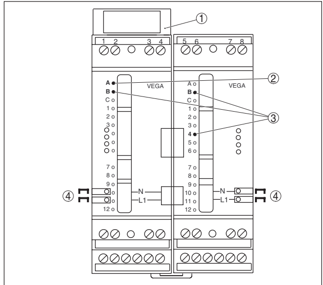
Рис. 2: Разъем VEGAMET 625
