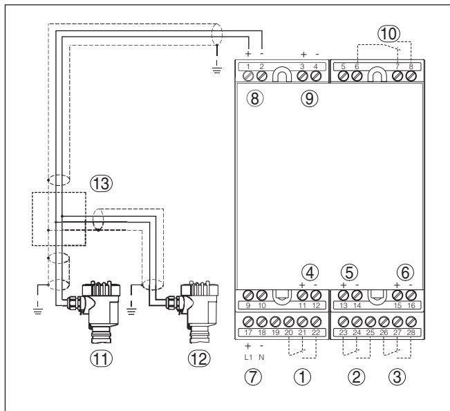
Рис. 3: Схема подключения VEGAMET 625 с двухпроводными датчиками
