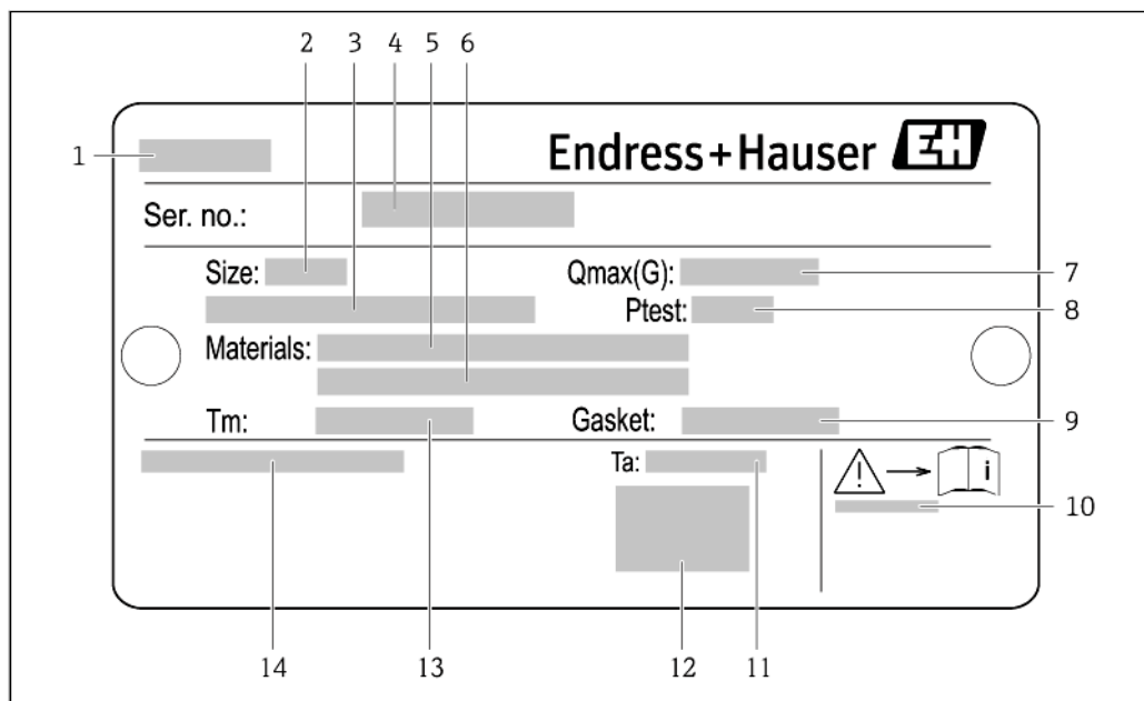
3 Пример шильды сенсора
