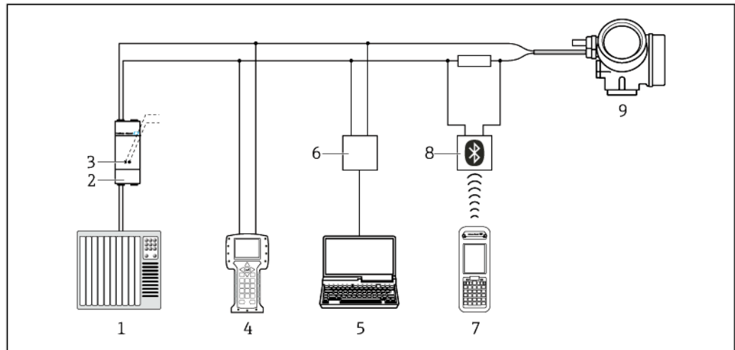
15 Варианты дистанционного управления по протоколу HART
