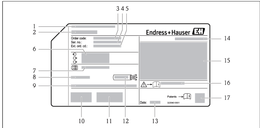
2 Пример шильды электронного преобразователя
