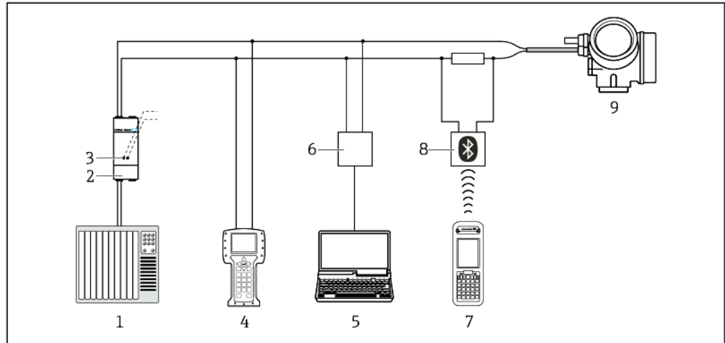
37 Варианты дистанционного управления по протоколу HART
