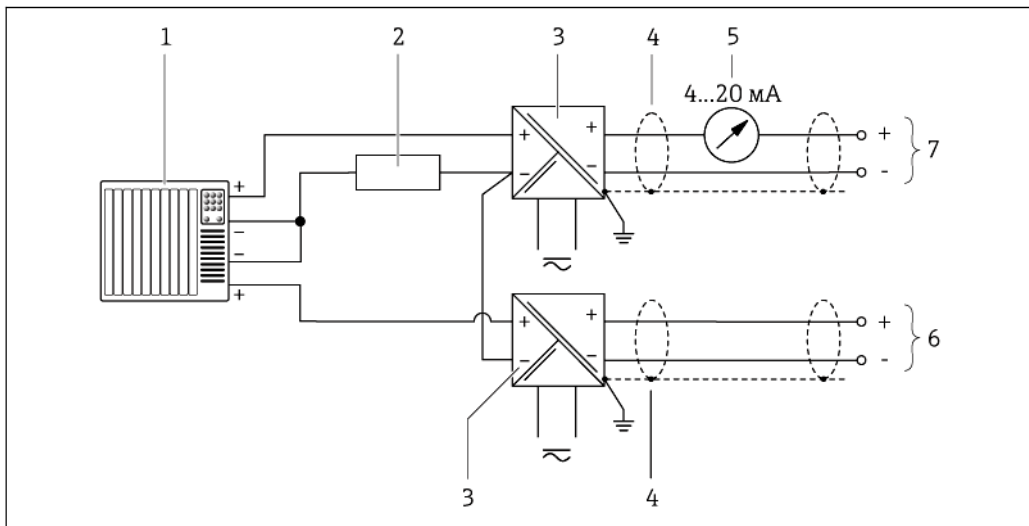
☛ 12 Пример подключения для входного сигнала HART с общим минусом
