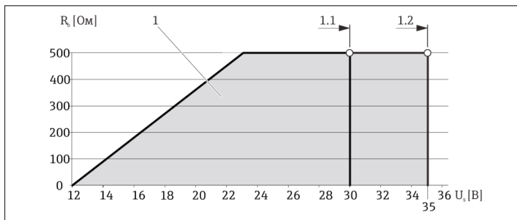
11 Нагрузка для компактного исполнения без местного управления
