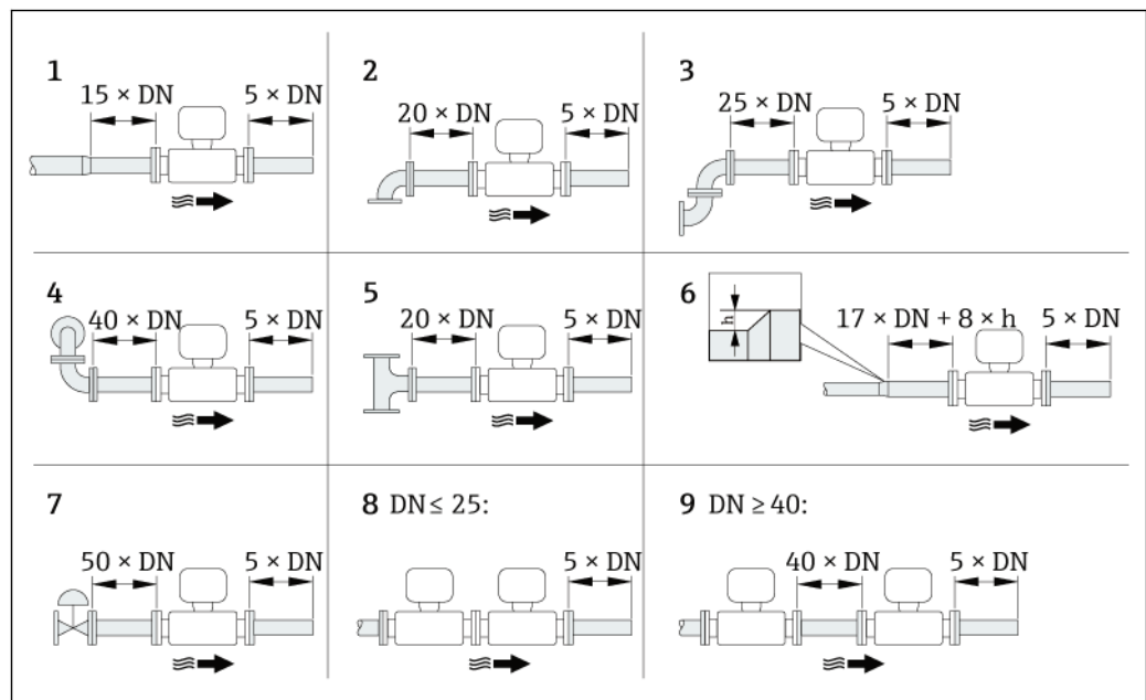
6 Минимальная длина входного и выходного прямых участков для различных вариантов препятствий
